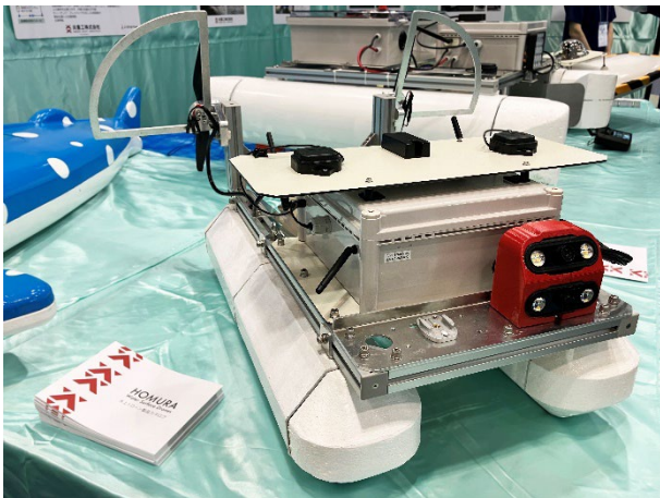
双胴艇タイプの水上演習ドローン
