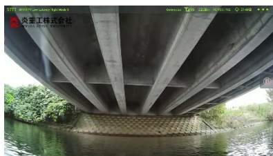
超小型水上ドローン『Swimmy Eye V1』を使った「見る」「撮る」「測る」例
